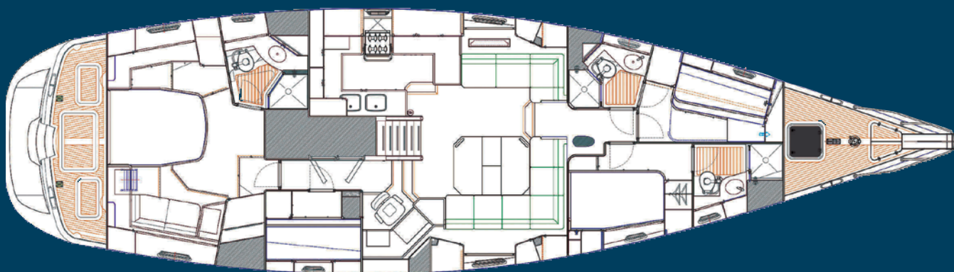
Sotto Vento interior layout
